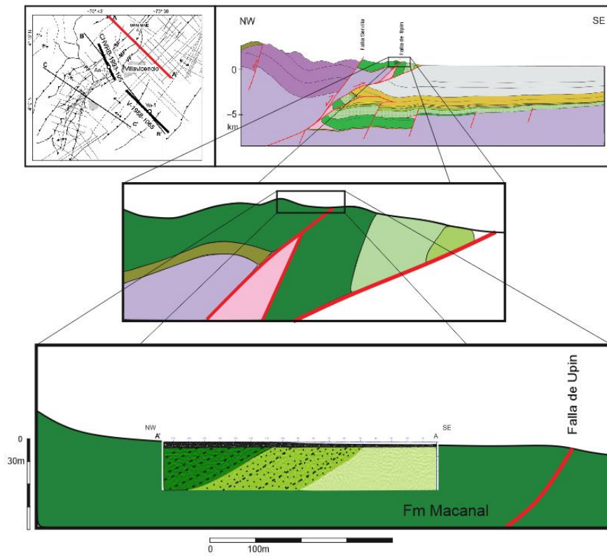
Figura 47. Imagen sísmica interpolada al modelo estructural propuesto por Parravano et al. (2015) tomado y modificado de: Parravano et al (2015).
