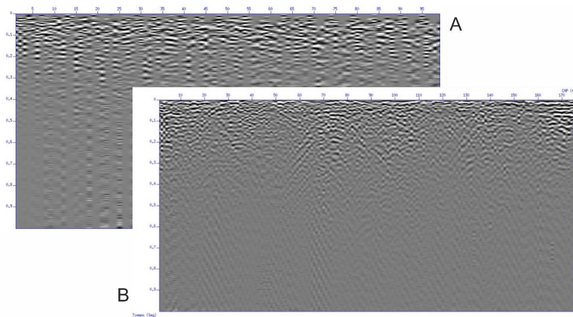
Figura 38. Comparación entre la Imagen sísmica con la corrección de estáticas aplicada (A) y posterior al proceso de apilamiento.
