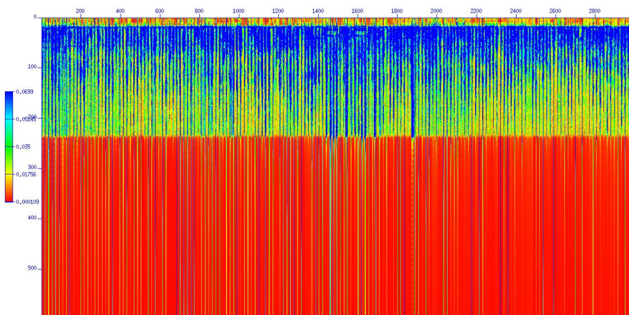
Figura 29. Dato sísmico en el dominio de la frecuencia luego de aplicar filtro Pasa-Baja
