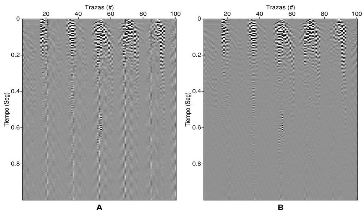
Figura 28. Comparación entre el dato con frecuencias altas (A) y el dato sin frecuencias altas (b) después de aplicar filtro Pasa-Alta.
