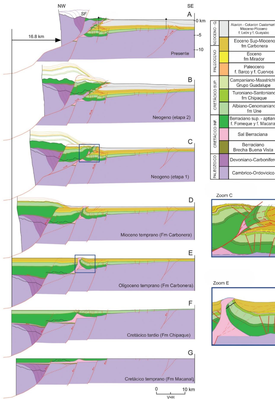
Figura 8. Modelo de evolución estructural local de la zona de estudio evidenciando la influencia de la tectónica salina en el desarrollo estructural del piedemonte llanero. Tomado y Modificado de Parravano et al (2015).
