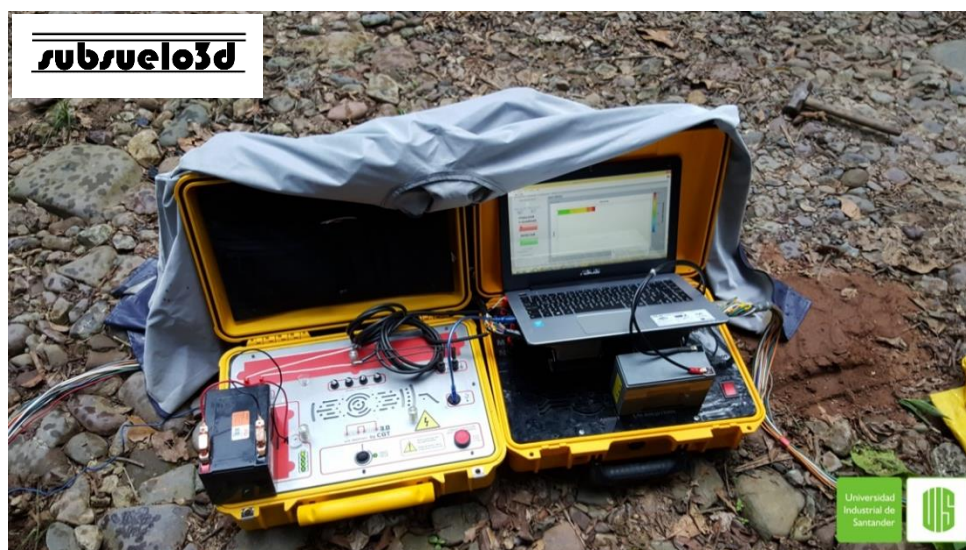
Figura 21. Equipo Geoelectrica utilizado para las tomografías eléctricas.
