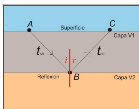
Figura 9. Diagrama de una trayectoria reflejada en el punto B, partiendo de A y detectada en C. Tomada y modificada de: Canales (2010).
