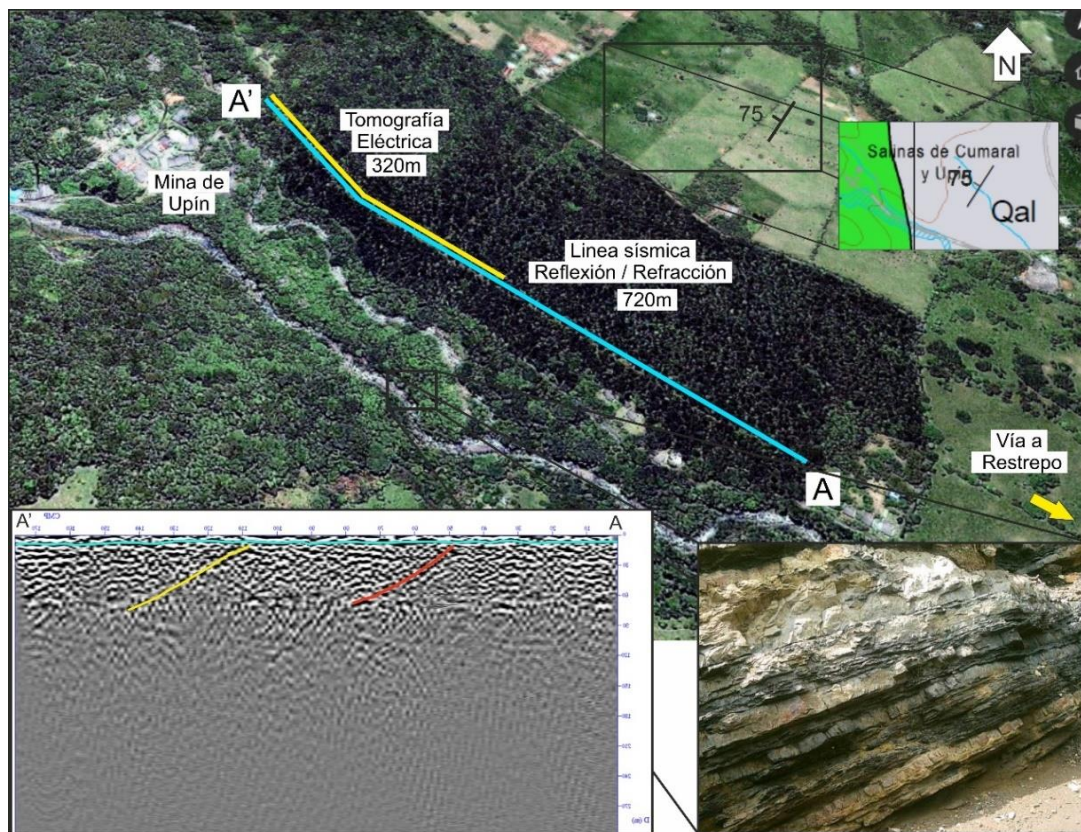
Figura 43. Integración de datos geológicos y estructurales que corroboran la naturaleza de los reflectores.
