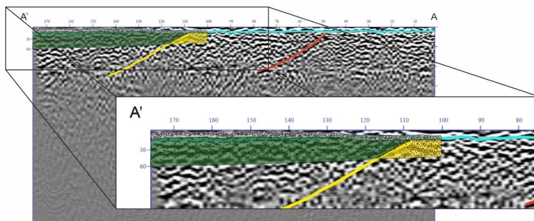
Figura 46. Interpolación de la imagen sísmica y la tomografía eléctrica interpretada
