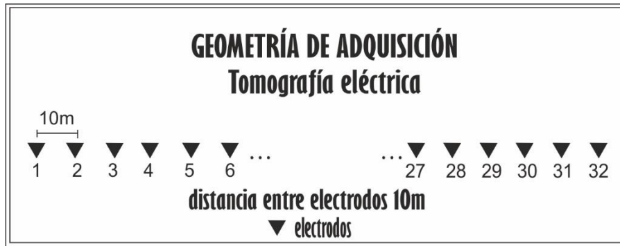
Figura 22. Geometría de adquisición para la tomografía eléctrica.
