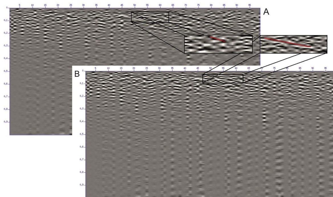
Figura 37. Dato sísmico con la ubicación real en el eje z de las trazas, posterior a la corrección de estáticas.
