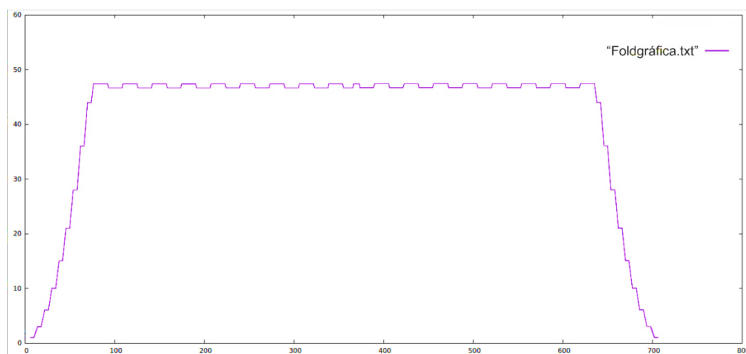
Figura 34. Cubrimiento sísmico determinado por el número máximo de trazas sísmicas en cada CMP.
