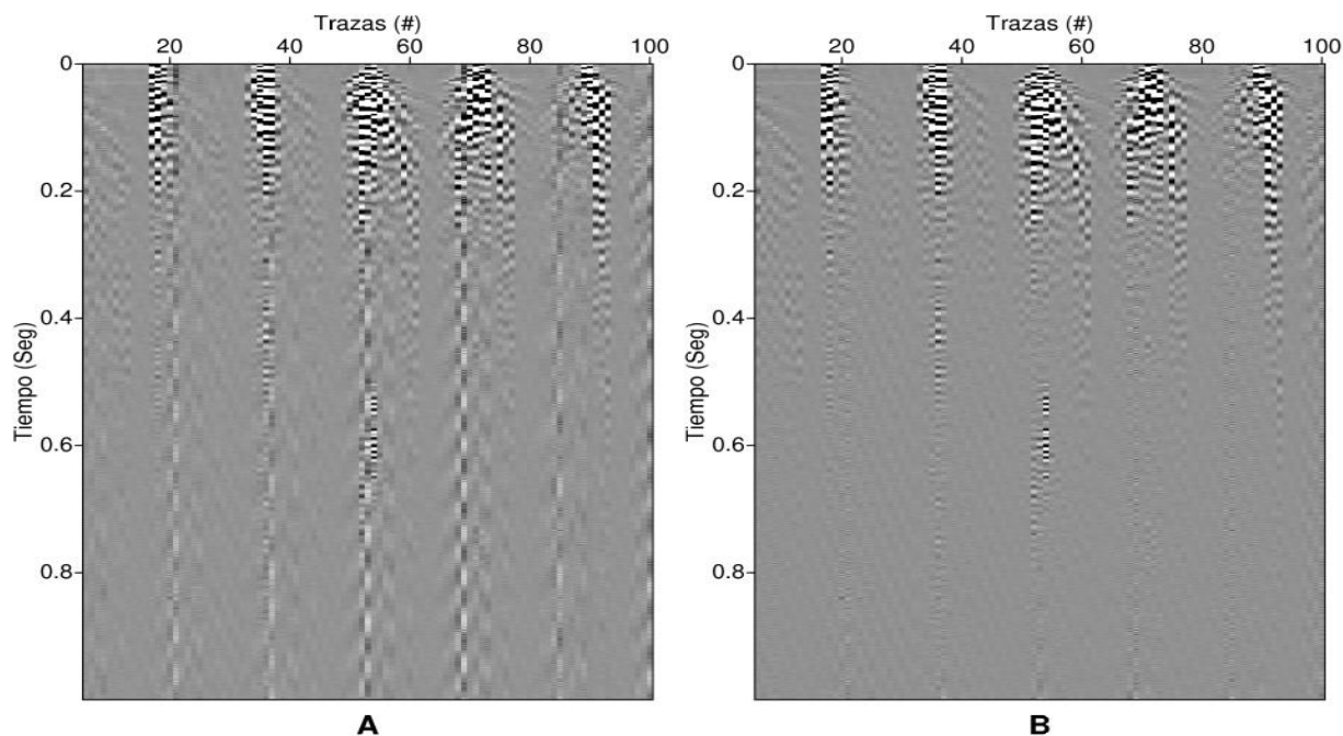
Figura 26. Comparación entre el dato con frecuencias bajas (A) y el dato sin frecuencias bajas (b) después de aplicar filtro Pasa-Alta.
